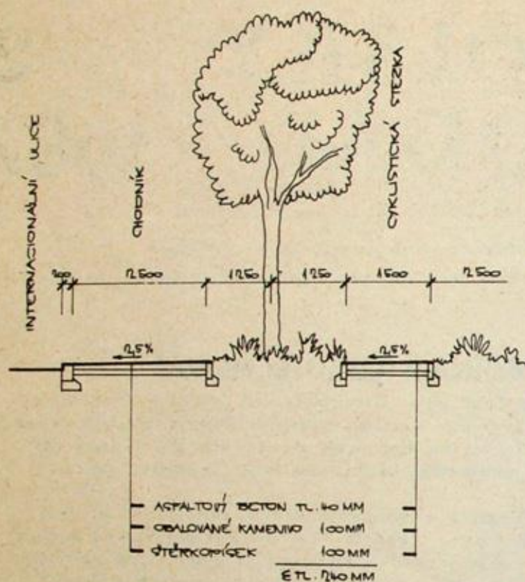
Obr. 2. Schéma úprav okolí vozovky v Internacionální ulici
