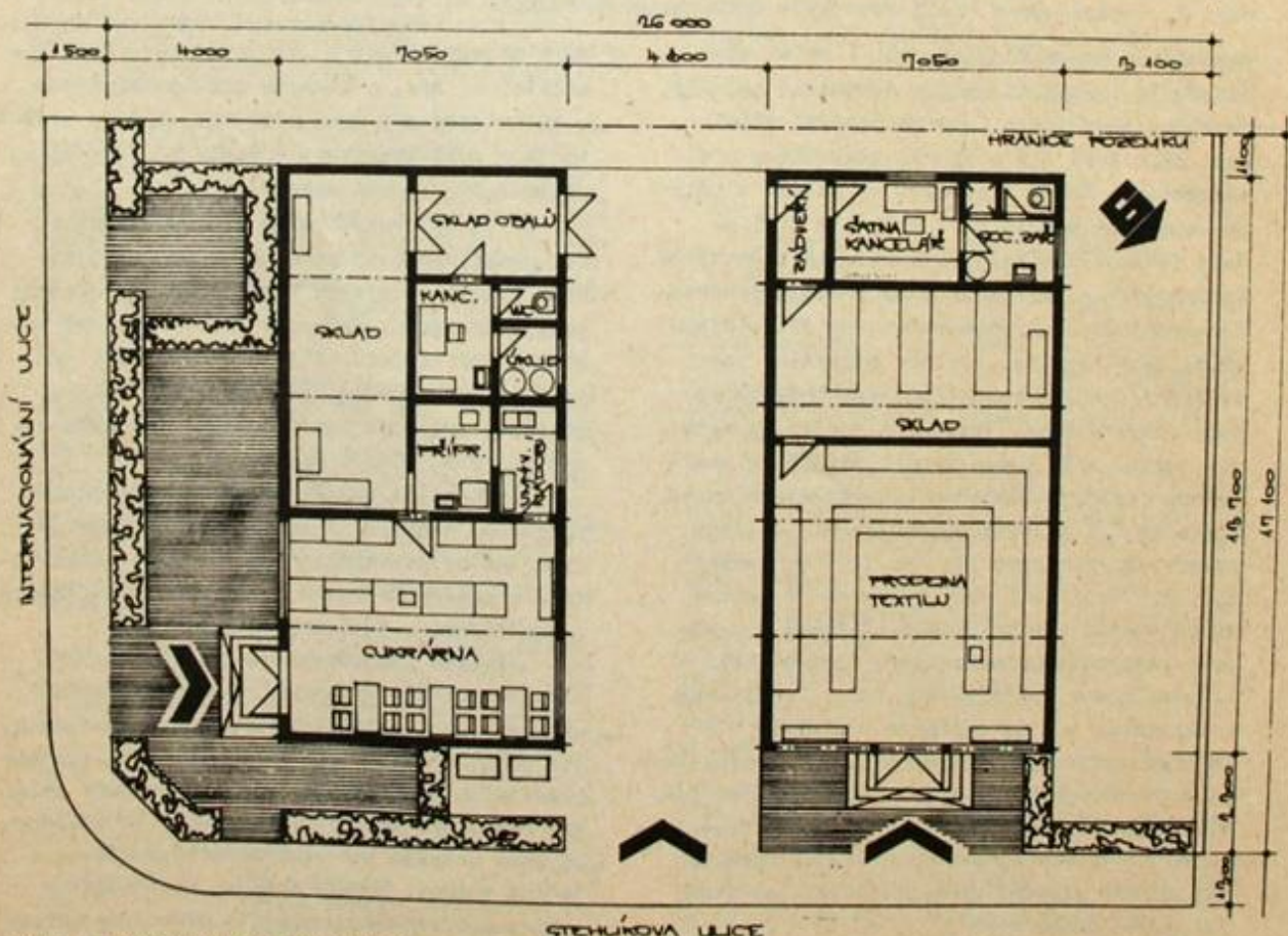
Schéma zástavby na rohu Stehlíkovy a Internacionální ulice
